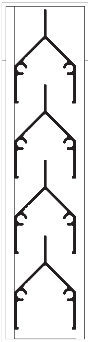
montagem dos perfis profiles assembly n31 437 e n30 253
