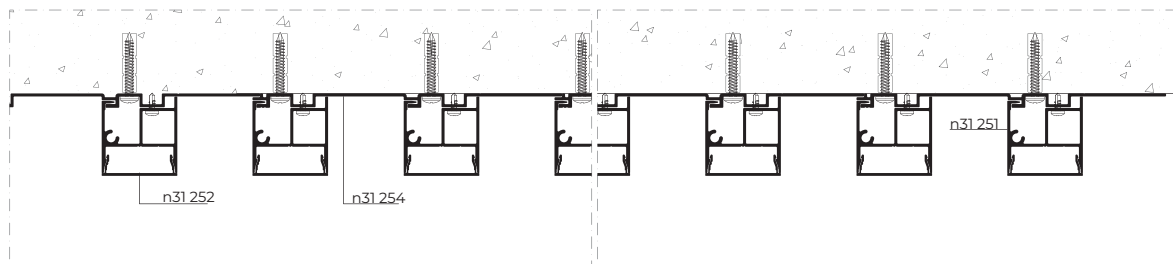
Corte B-B' Section B-B'
