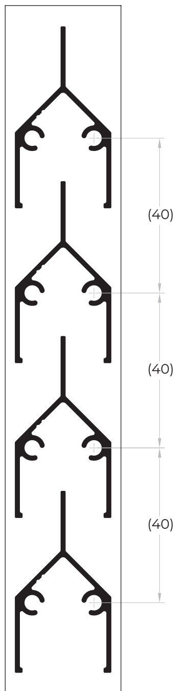
montagem dos perfis profiles assembly n31 438 e n30 150
