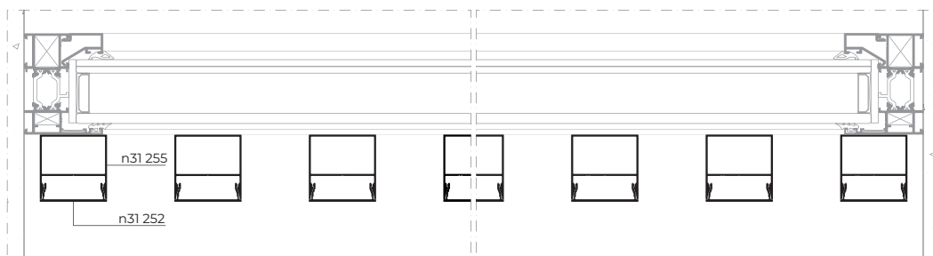
Corte B-B' Section B-B'
