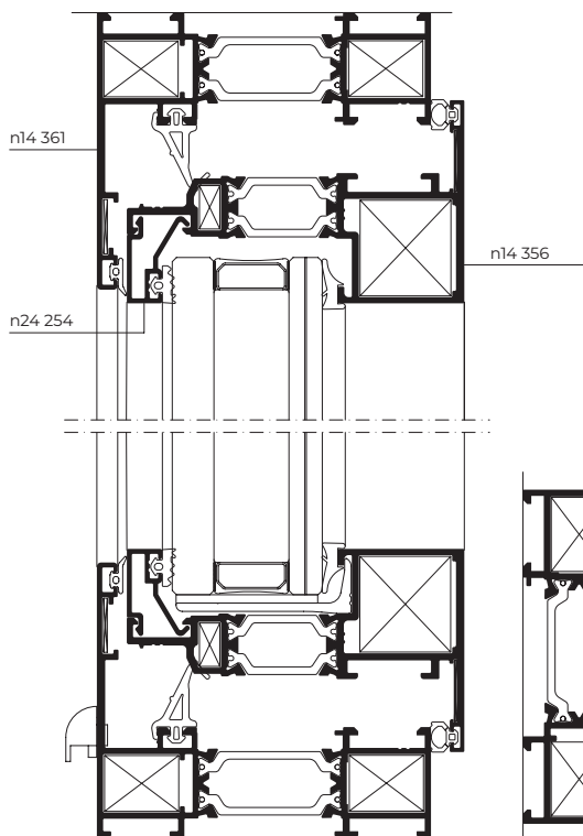
Corte A-A' Section A-A'
