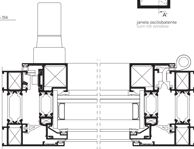
Corte B-B' Section B-B'
