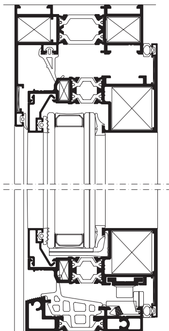
Corte A-A' Section A-A'
