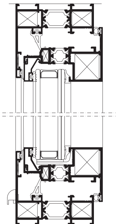
Corte A-A' Section A-A'
