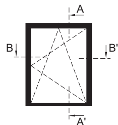
janela oscilobatente com soleira turn tilt window with sill
