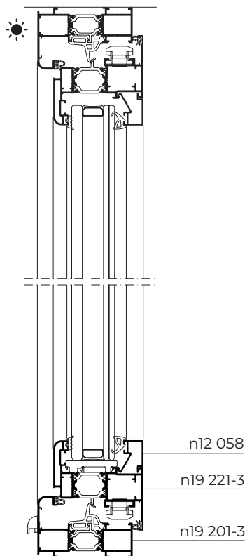
Corte A-A' Section A-A'
