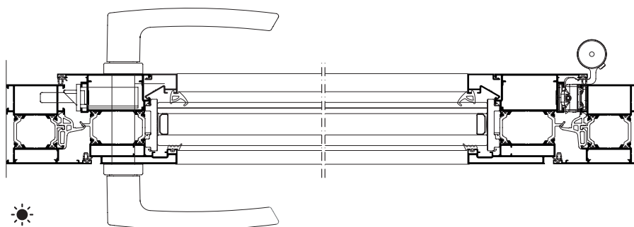
Corte B-B' Section B-B'
