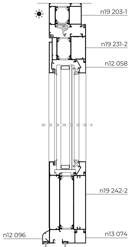
Corte A-A' Section A-A'
