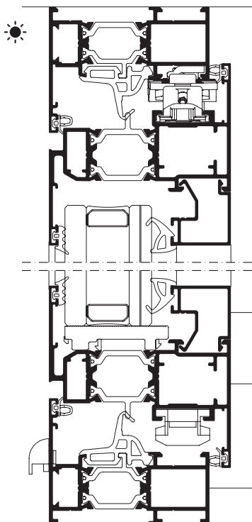
OSCILOBATENTE 2 FOLHAS 2 SASHES TILT AND TURN WINDOW
