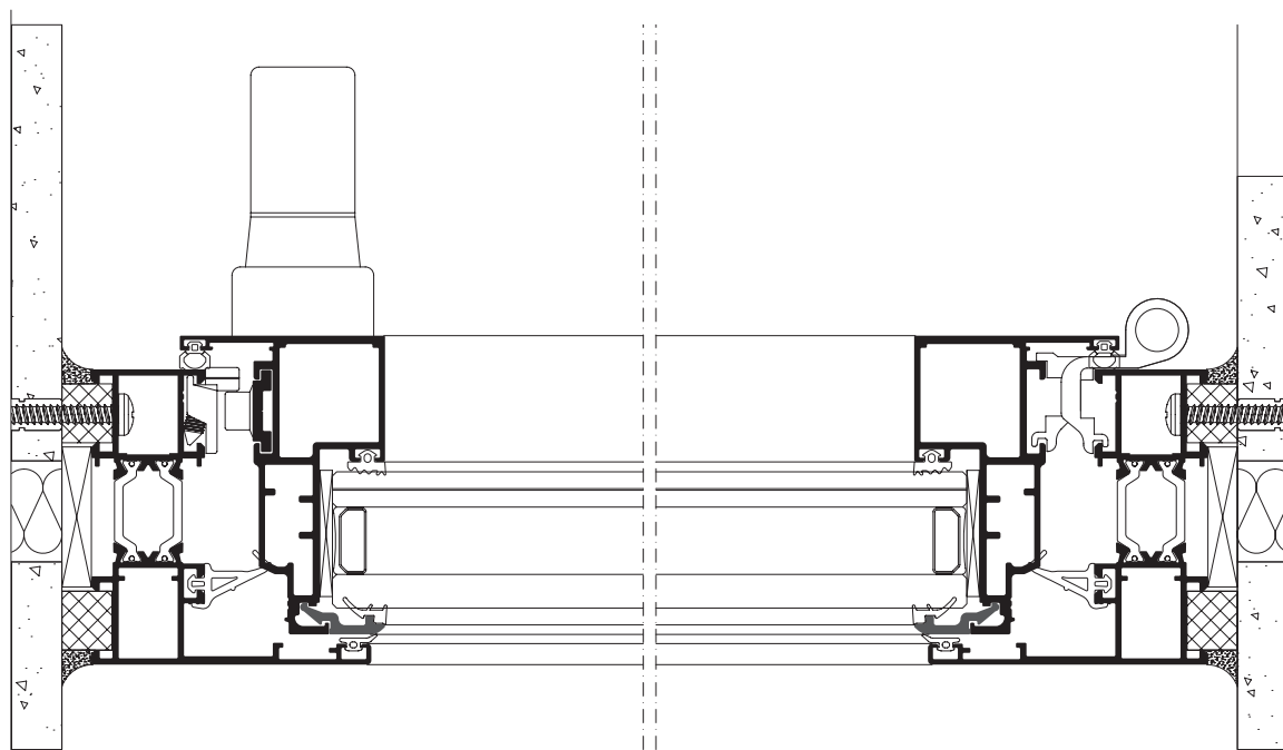
Corte B-B' Section B-B'
