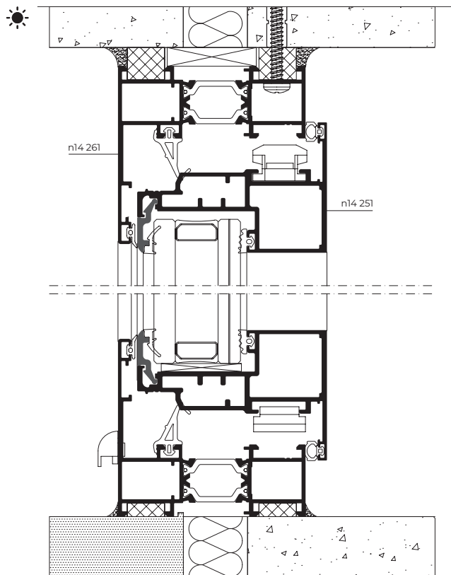
Corte A-A' Section A-A'
