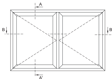
janela de batente 2 folhas 2 sashes side-hung window
