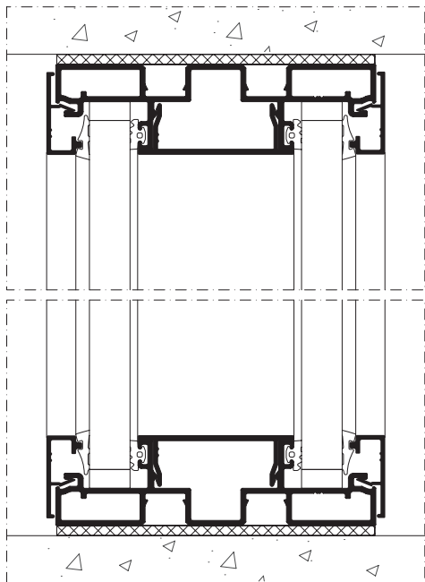
Corte A-A' Section A-A'
