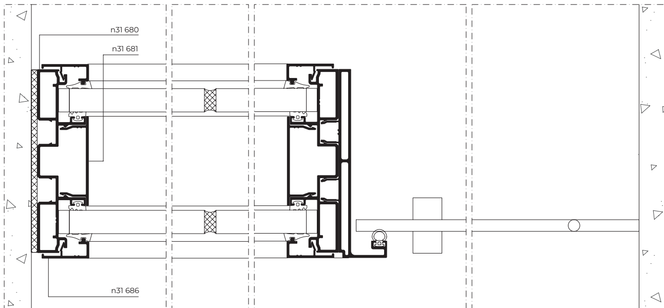
Corte B-B' Section B-B'
