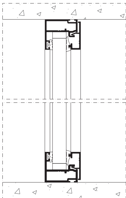
Corte A-A' Section A-A'
