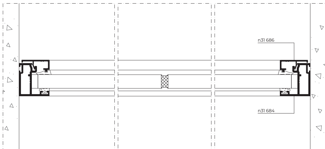
Corte B-B' Section B-B'
