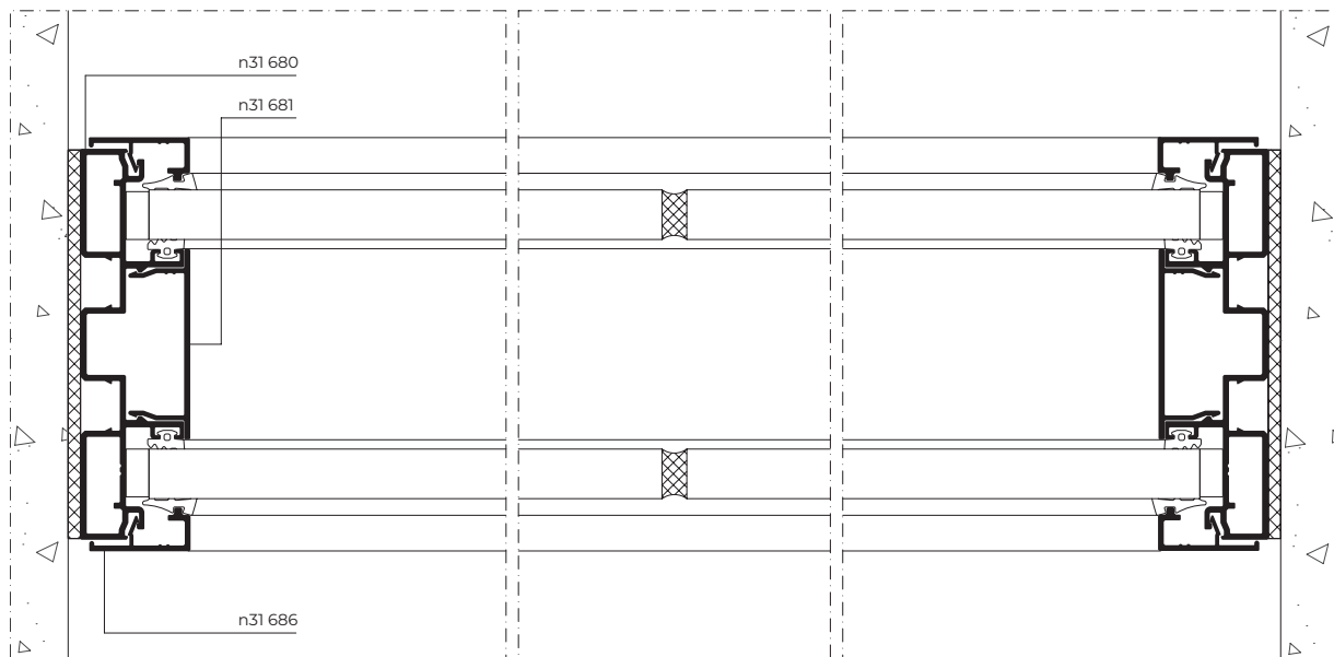
Corte B-B' Section B-B'
