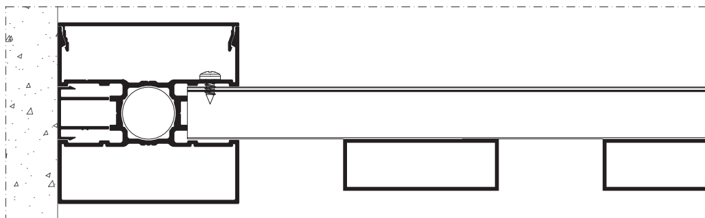
Corte B-B' Section B-B'
