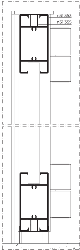
Corte A-A' Section A-A'
