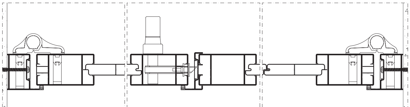
Corte B-B' Section B-B'
