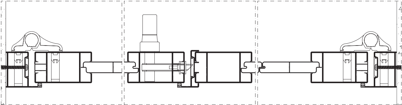
Corte B-B' Section B-B'
