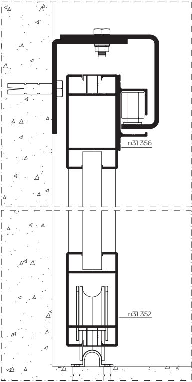
Corte A-A' Section A-A'
