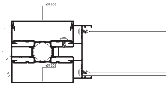
Corte B-B' Section B-B'
