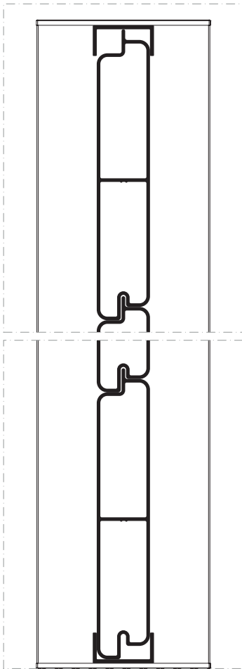
Corte A-A' Section A-A'
