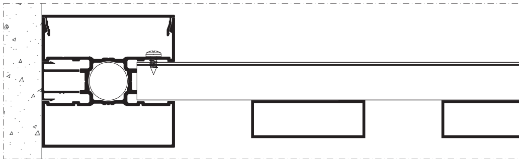
Corte B-B' Section B-B'
