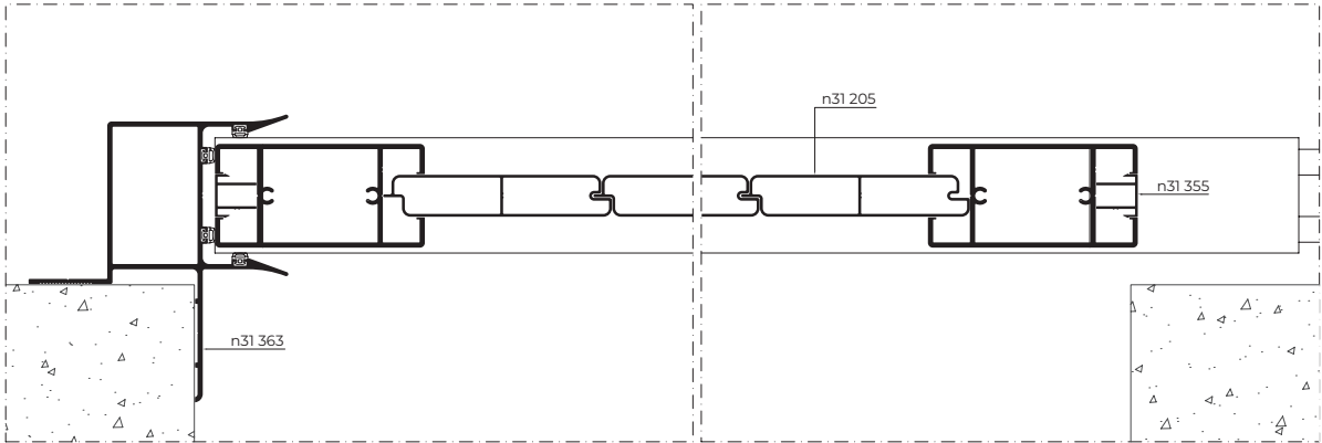
Corte B-B' Section B-B'
