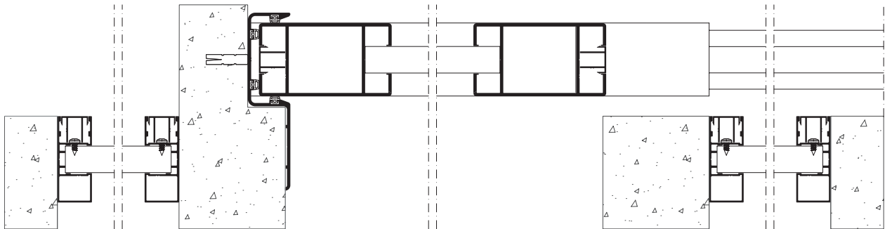
CORTE: B-B' SECTION: B-B'
