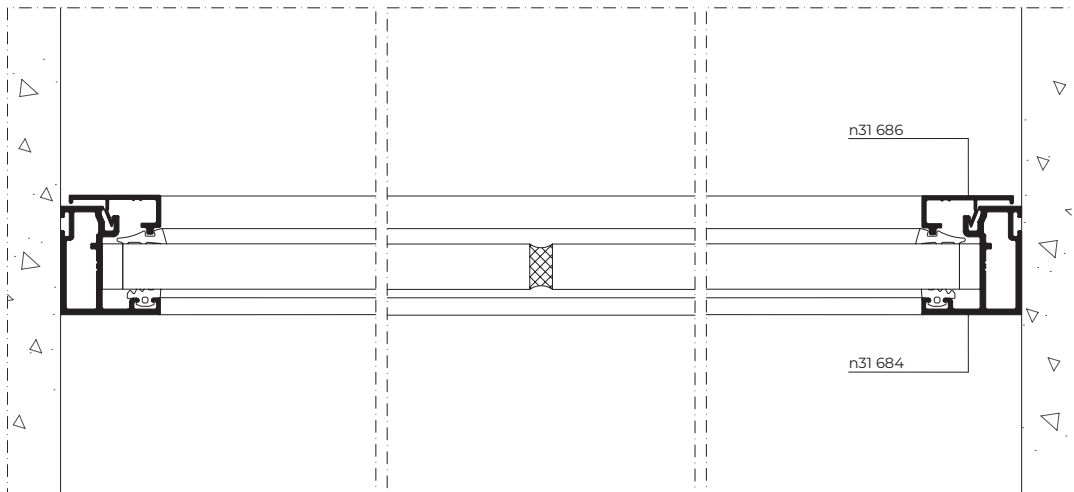
Corte B-B' Section B-B'
