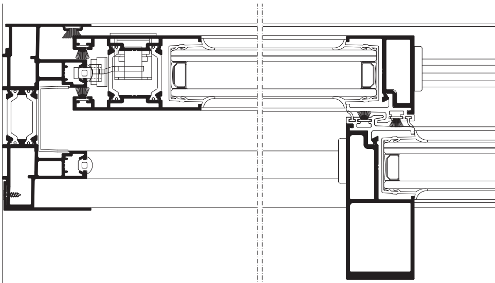
Corte A-A' Section A-A'
